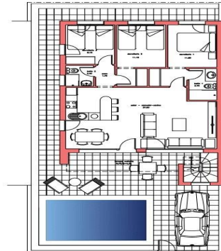
PLANTA BAJA SUP. UTIL : 79,85 M2. SUP. CONSTRUIDA: 94,00 M2. SUP. DE PARCELA NETA: 200,00 M2.
